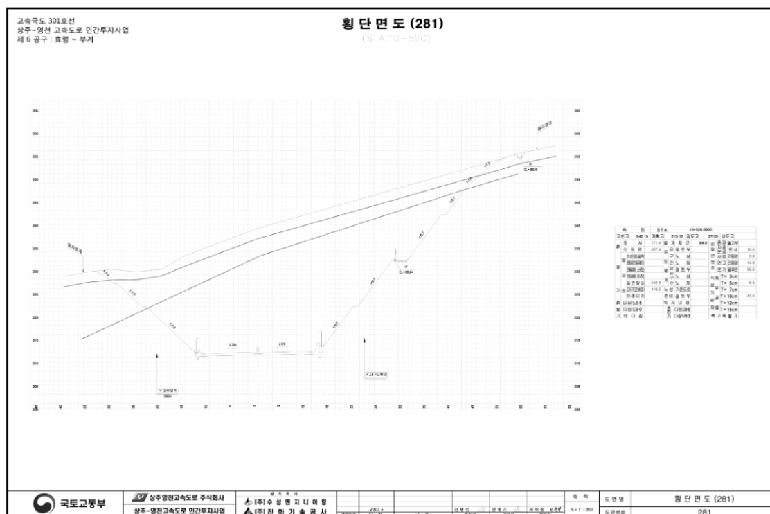
【그림 38.4】 표준형단면도
